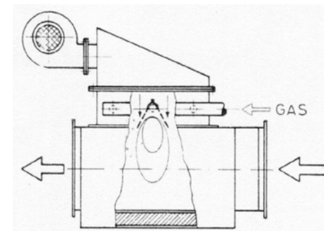
MIXBLOC EE EXTERNAL BURNER & COMBUSTION AIR FAN
